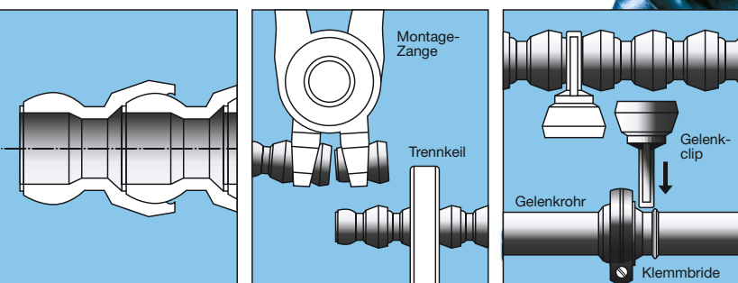
gleichbleibender Querschnitt
